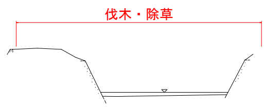
標準断面図 (蛇池川)
